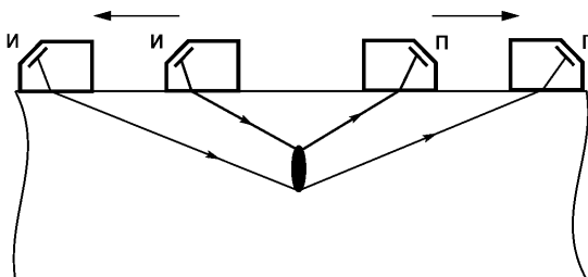
Рисунок 5 — Дифракционный
